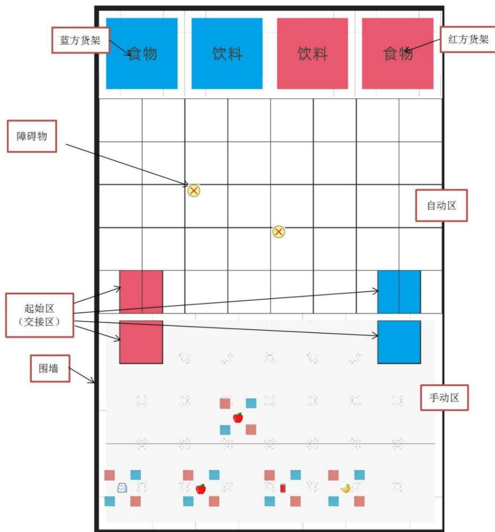
图1 模拟物流仓库场地示意图
