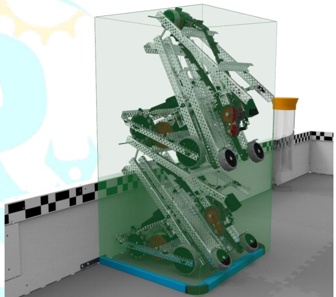
图 SC4-2：两台机器人停泊均有效，因为这两台机器人都满足以上所有标准
